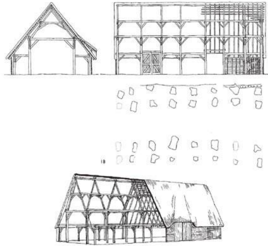
Oost-souburg: huisplattegronden
